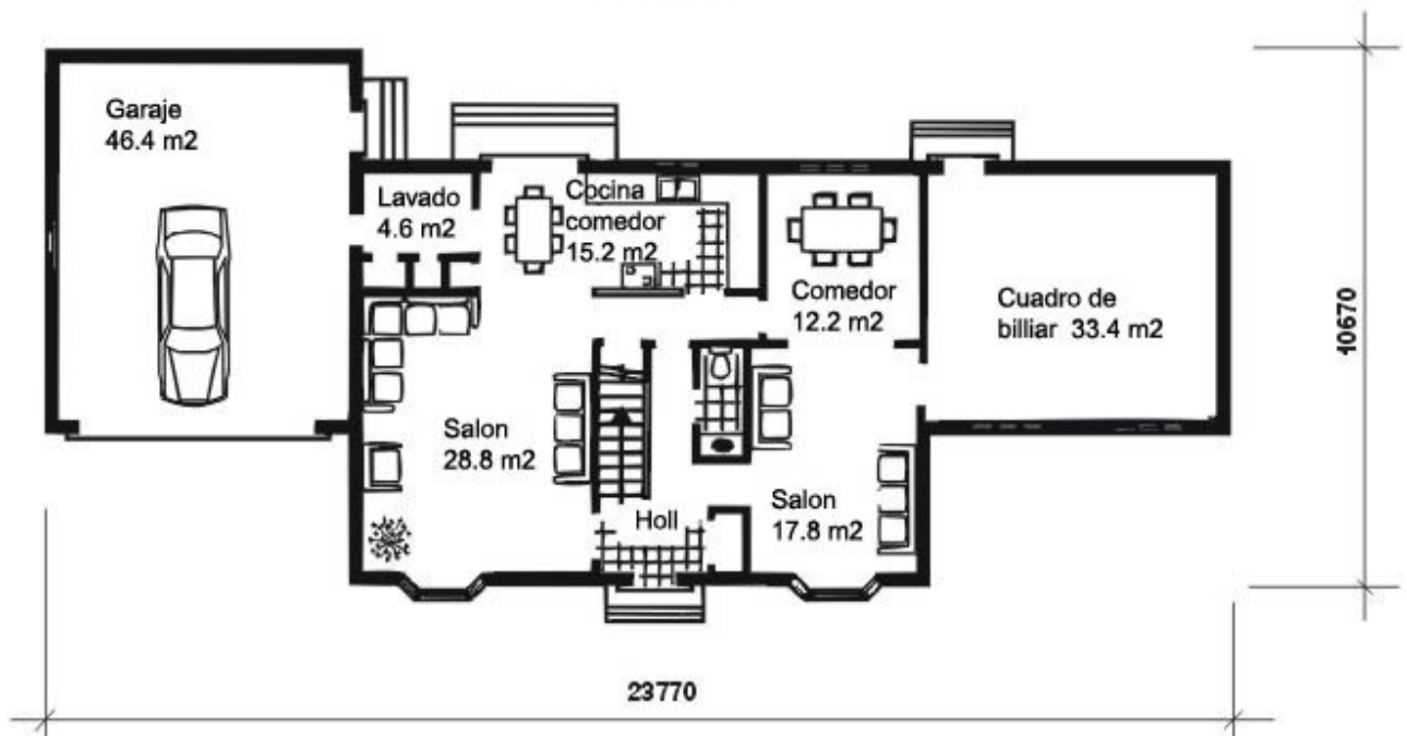
Planta baja
