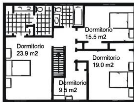
Primera planta
